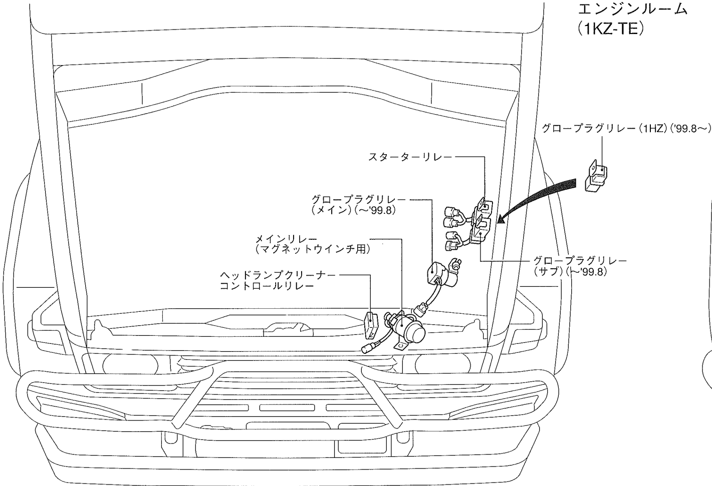
エンジンルーム (1HZ, 1PZ)
