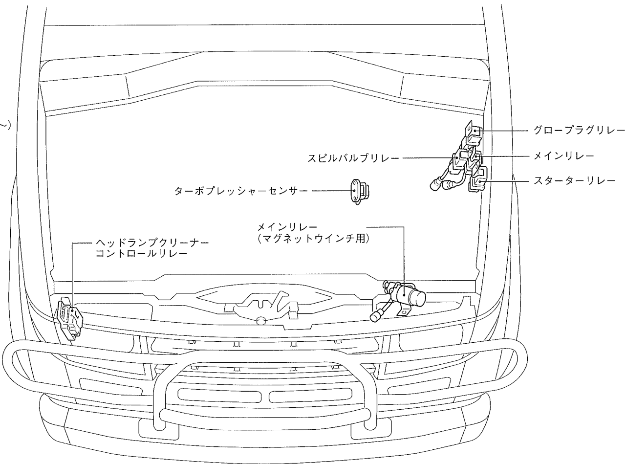
エンジンルーム (1KZ-TE)
